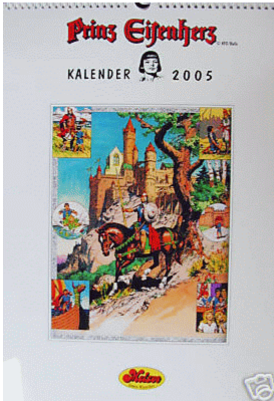
Abb.1: Kalender 2005 (Auszug)
